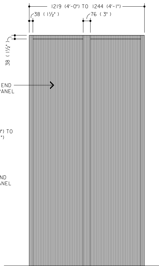
ELEVATION E
